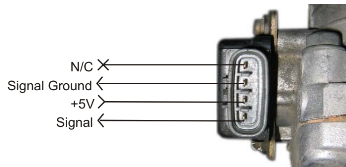
Figure S01.1 - Subaru TPS Pinout
